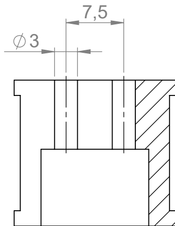
SCHNITT A-A
